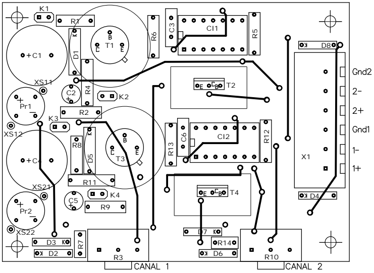
Top layer / Component side - Fata de sus / Partea cu piese
