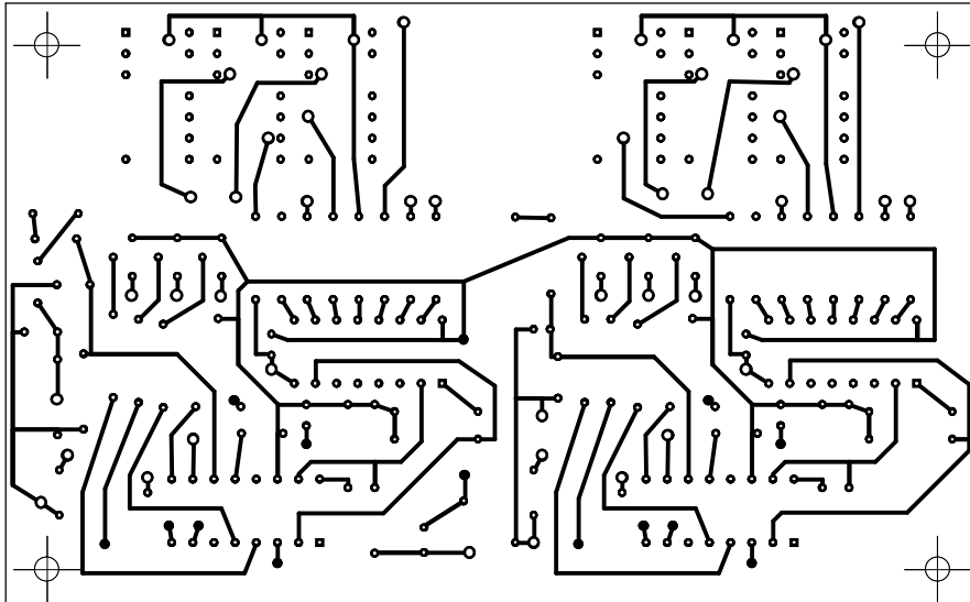
Modul voltmetru si ampermetru (fata de jos, in oglinda)
