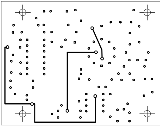
Modul stabilizator tensiune (fata de sus)
