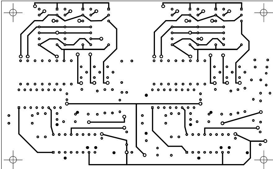
Modul voltmetru si ampermetru (fata de sus)
