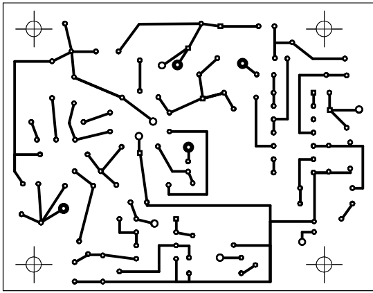
Modul stabilizator tensiune (fata de jos, in oglinda)
